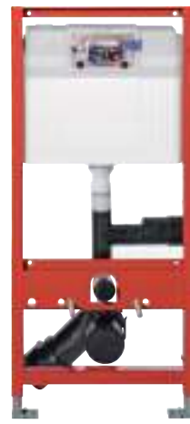
TECEprofil 9300303 Inštalčný modul s nádržkou UNI pre WC, výška 1,12 m s pripojením pre odsávanie zápachu
